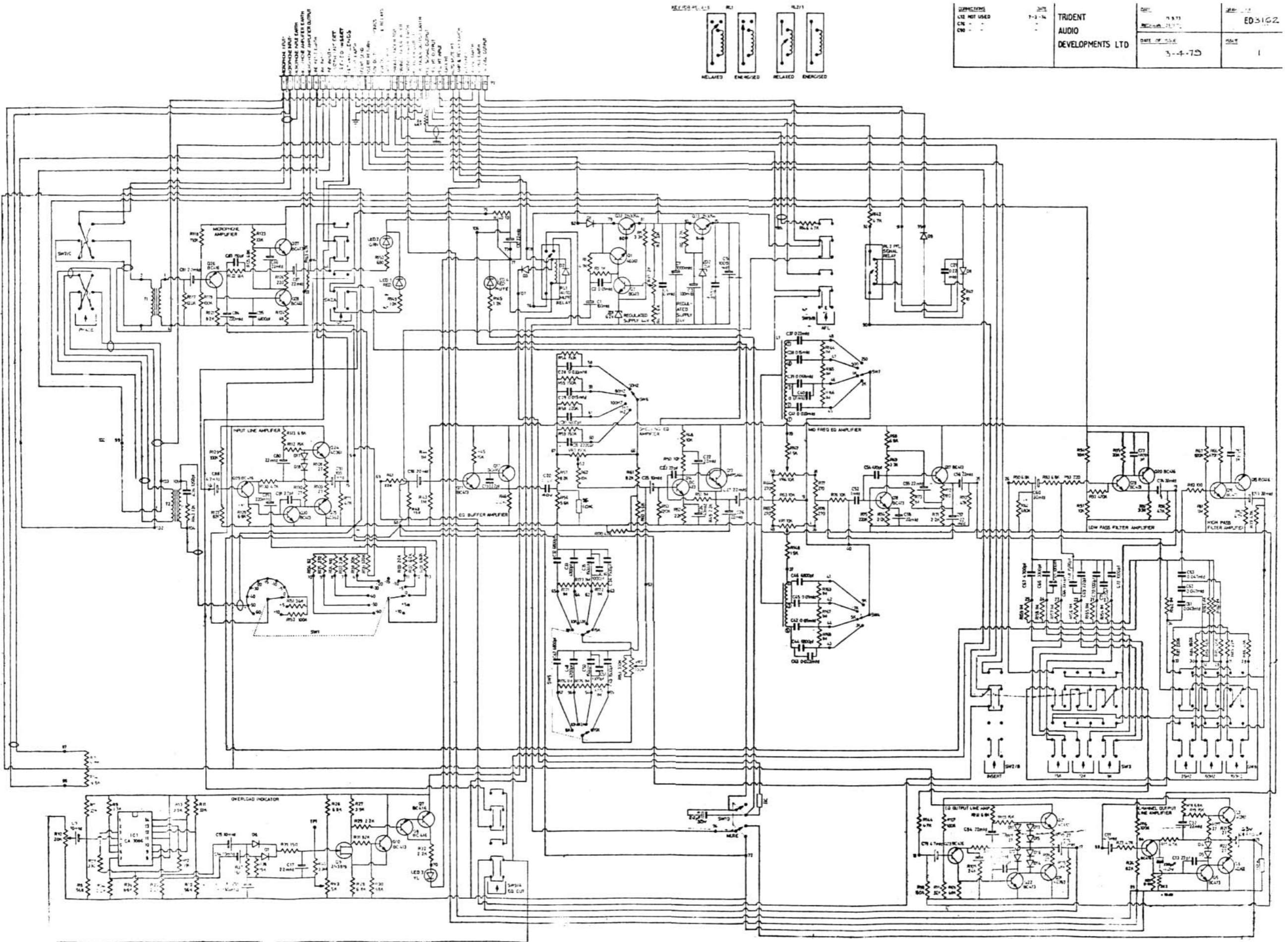
Trident A-range channel module
